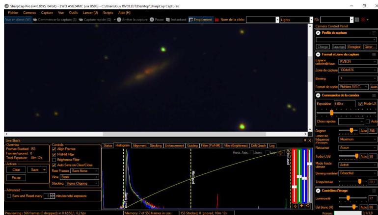
M82 Galaxie du cigare
